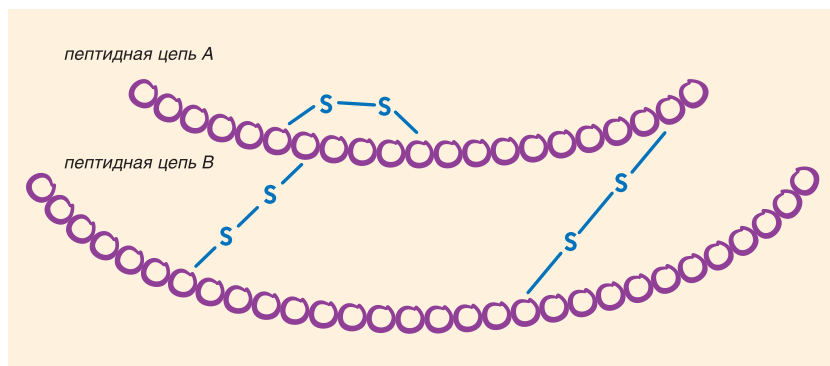
Структура инсулина
